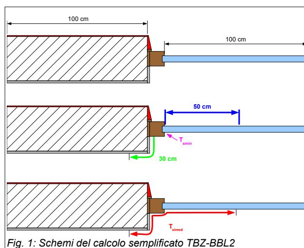
Fig. 1: Schemi del calcolo semplificato TBZ-BBL2
